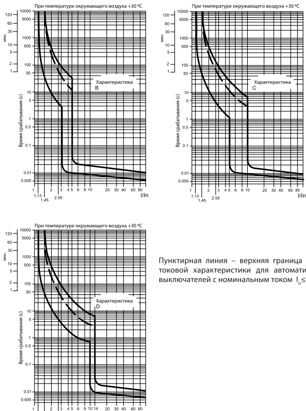
Рисунок 1. Время-токовые характеристики
